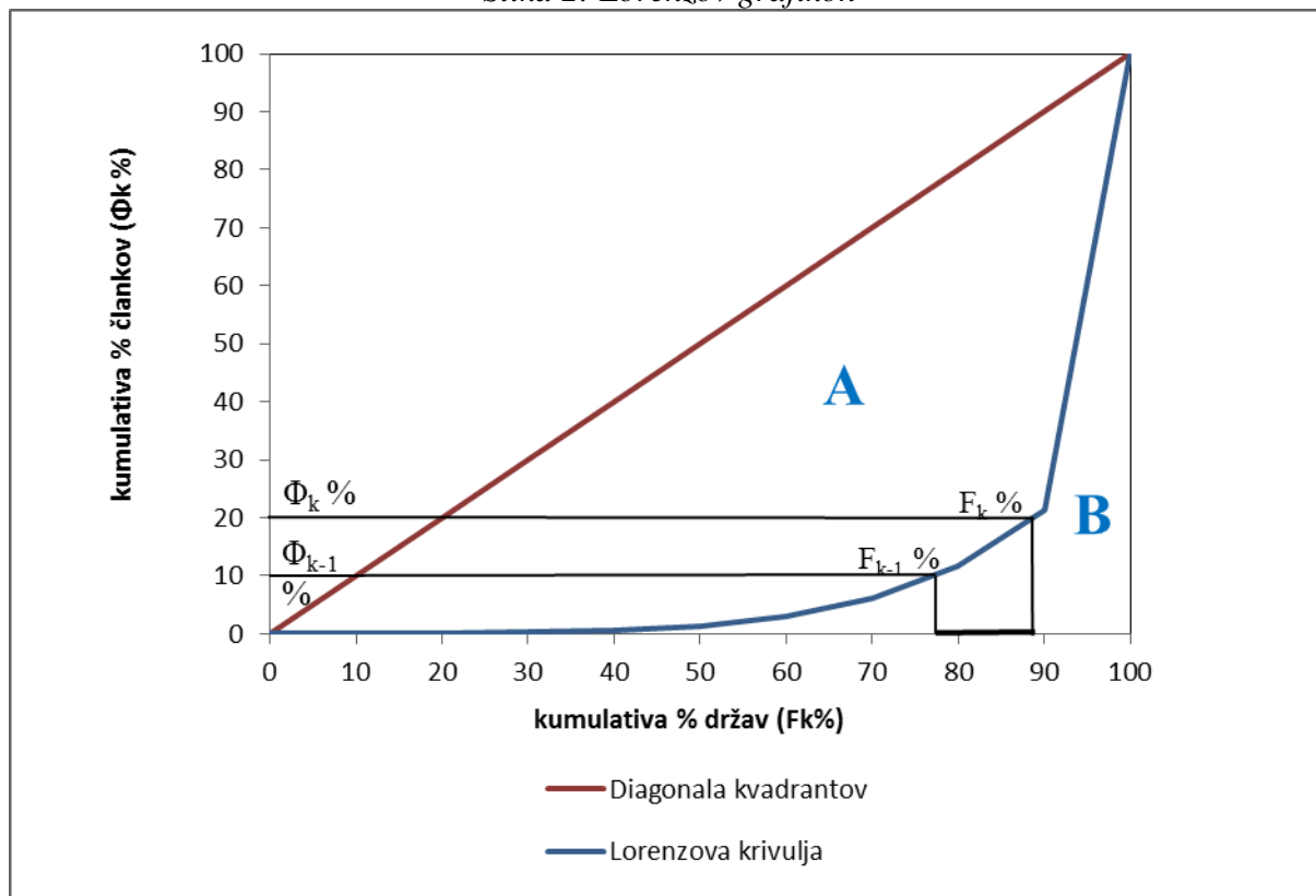
Slika 2: Lorenzov grafikon
