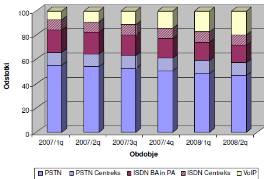
Slika 1: Deleži telefonskih priključkov po tehnologijah
