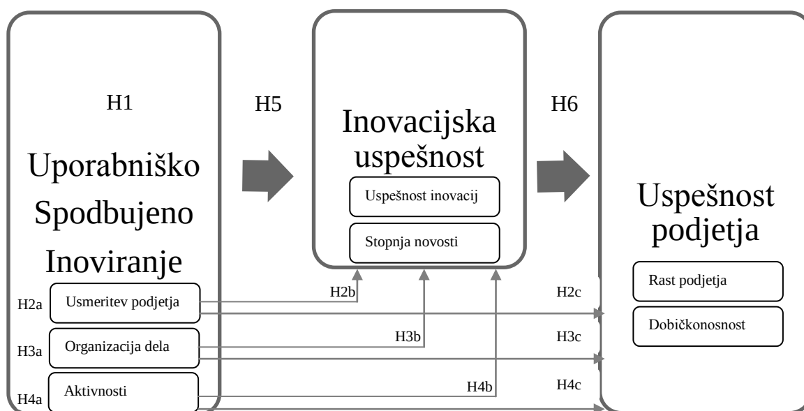
Slika 24: Konceptualni model
