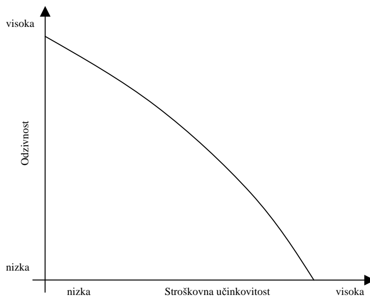
Slika 15: Stroškovno-odzivnostna meja
